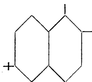
\beta Naphthohydrochinon- sulfosäure Witt. Ber. 14. 3154.
